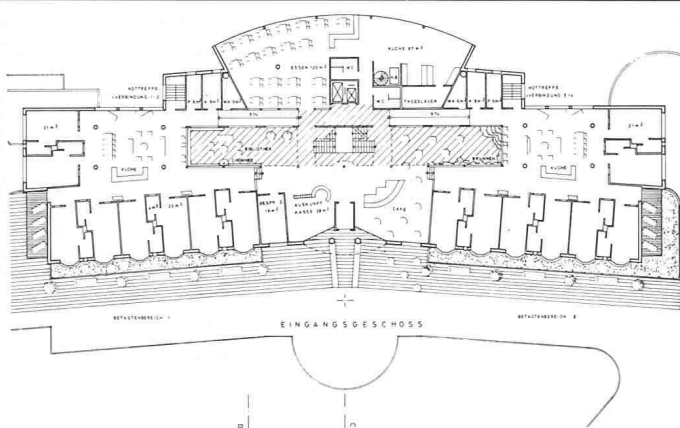
Grundriss Erdgeschoss 1:900
