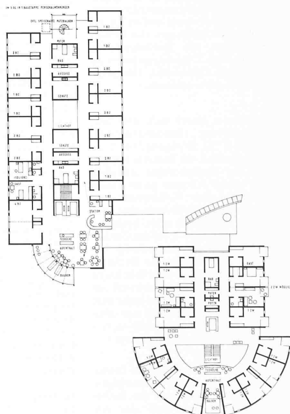
1.-3. Obergeschoss
