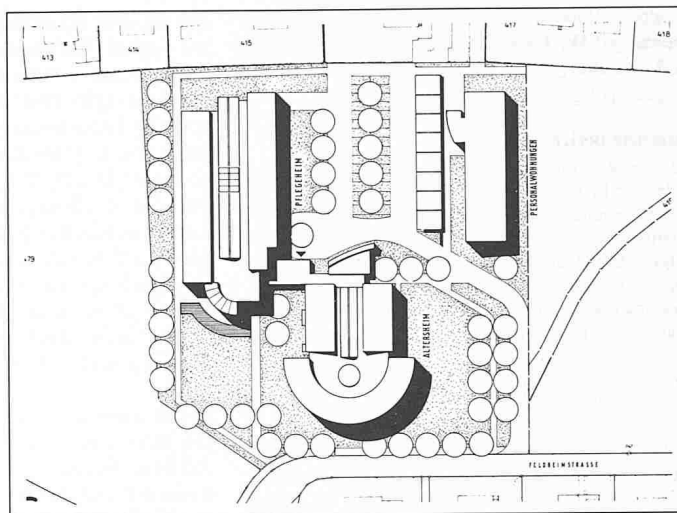
Lageplan 1:2000
