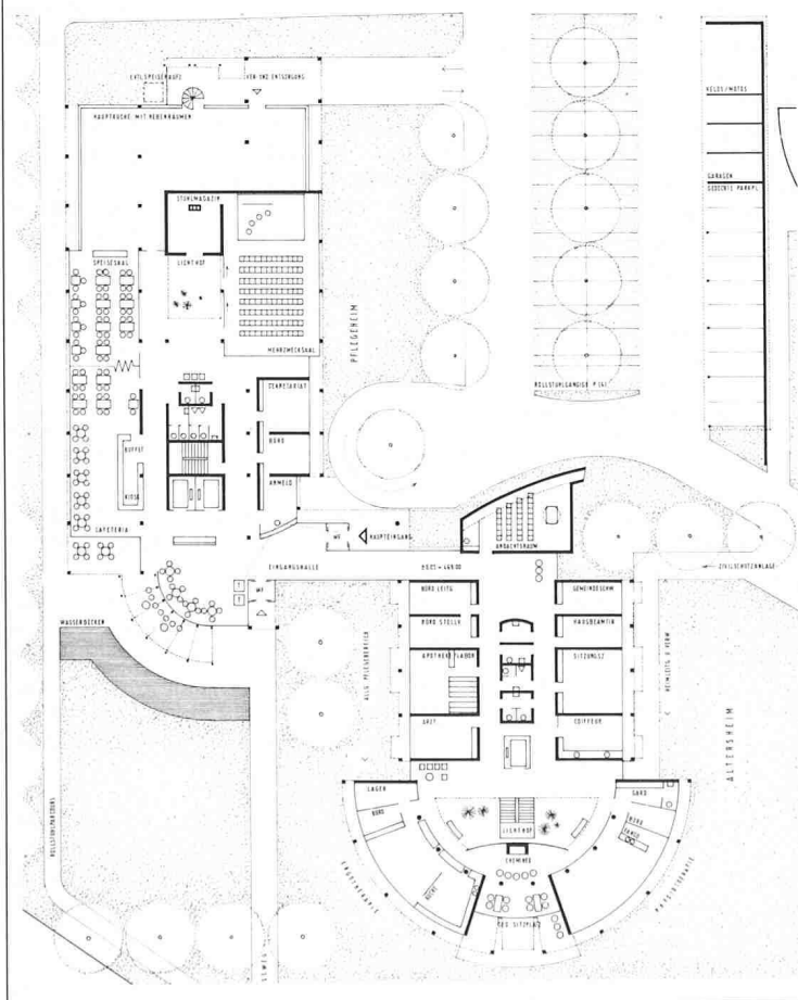
Grundriss Erdgeschoss 1:800
