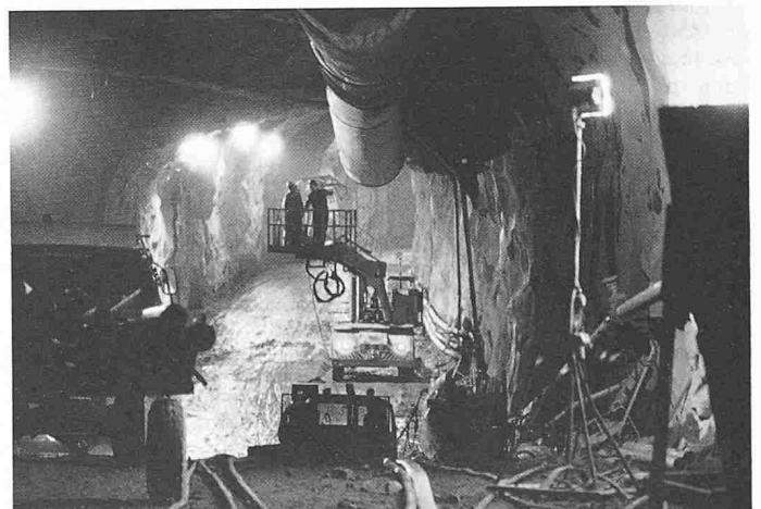
Bild 2. Bau des unterirdischen Endlagers für schwach- und mittlerradioaktive Abfälle in Forsmark (Schweden). Das Endlager soll 1988 den Betrieb aufnehmen und in den späten neunziger Jahren erweitert werden
