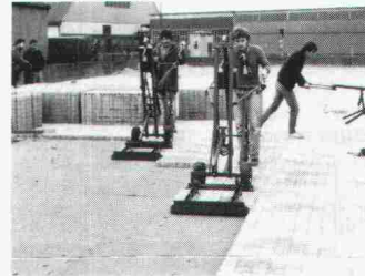
Uni-Verlegegerät
