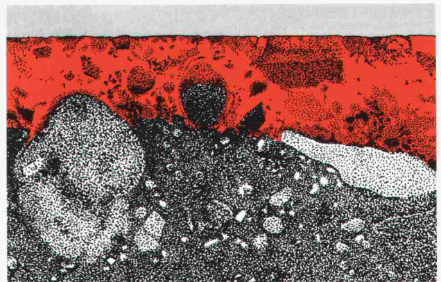
Sichtbare Eindringtiefe einer PERLTEX-Beschichtung auf dichtem Beton PC 300. Dargestellt in natürlicher Grösse.
