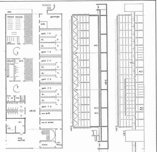
Untergeschoss
