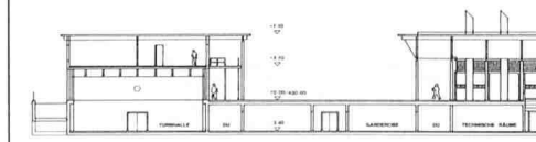
Schnitt
