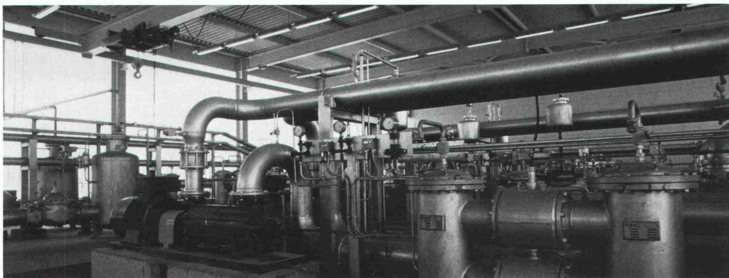
Brennstoff-Einlagerungspumpstation
