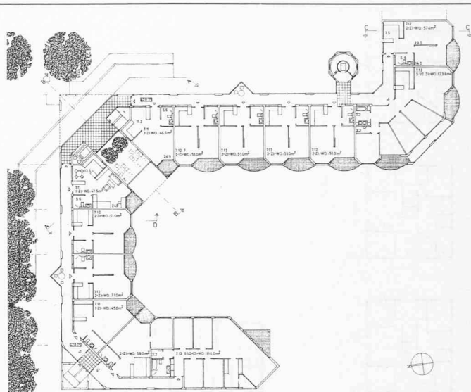
Grundriss 1.-3. Obergeschoss
