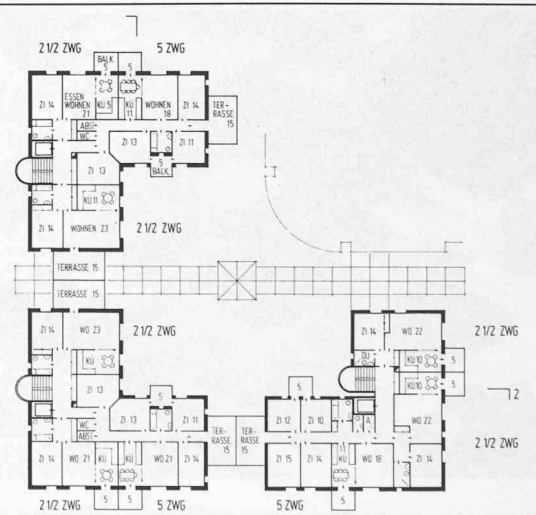
Grundriss 1./3. Obergeschoss
