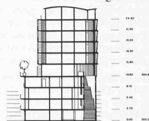
2. Obergeschoss Querschnitt
