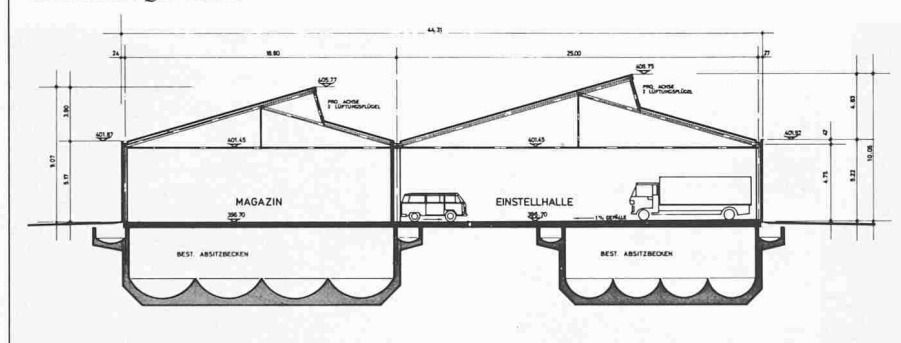
Einstellhalle. Querschnitt
