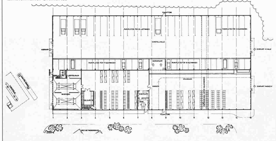
Einstellhalle. Grundriss
