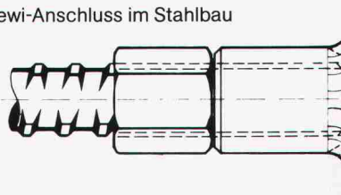
Gewi-Anschluss im Stahlbau
