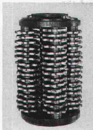
Hartmetall-Lamellen: zum Aufrauen und zum Entfernen von Farben, Überzähnen usw.
