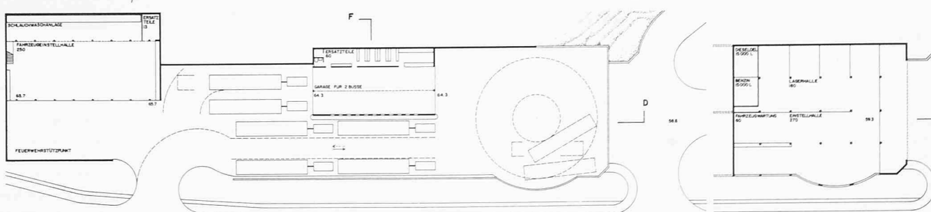
Grundriss Feuerwehrtützpunkt und Busgarage 1: 900
