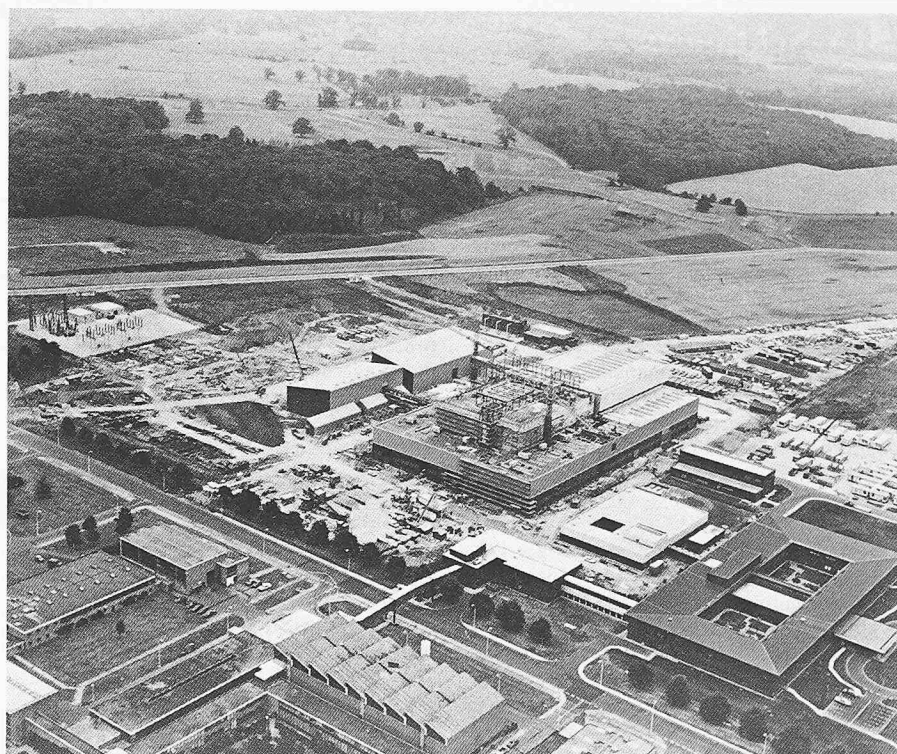
Die Bauarbeiten am europäischen Fusionsexperiment Jet in Culham sind so weit fortgeschritten, dass mit der Inbetriebnahme 1983 zu rechnen ist. In der Bildmitte, noch im Bau, die Experimentierhalle von Jet
