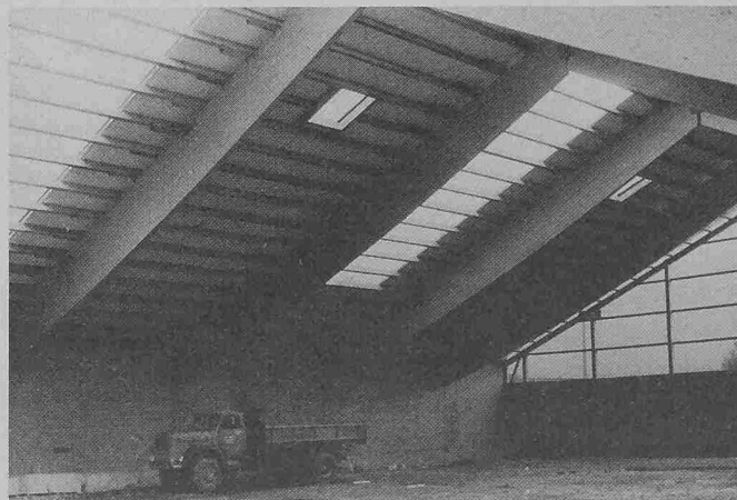
Tennishalle Bad Ragaz mit Gantner Isolier-Unterdach
