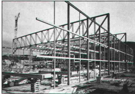
Stahlkonstruktion einer Lager- bzw. Einfeldhalle für Material und Fahrzeuge
