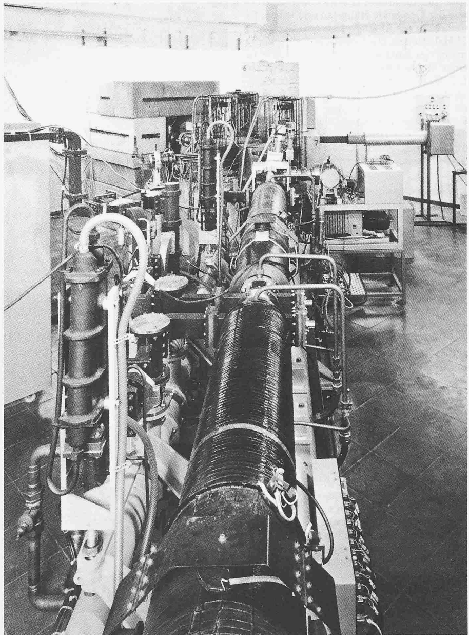
35 MeV-Linearbeschleuniger der BAM
