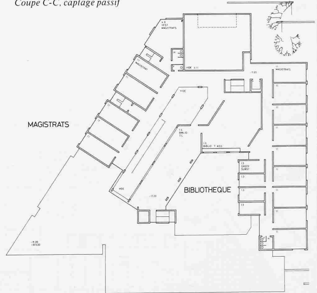
Plan du 4e étage
