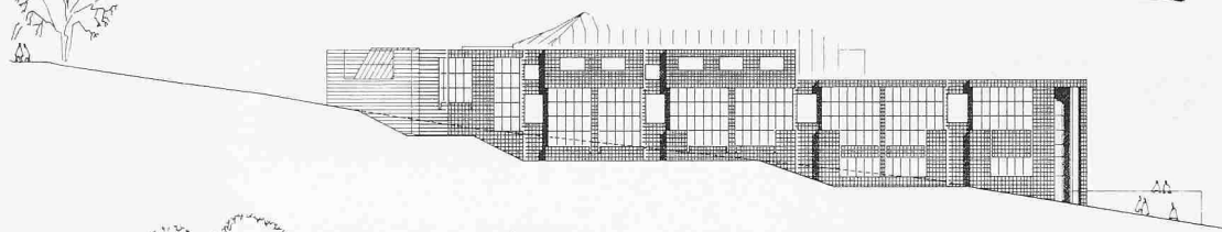
Façade sud-ouest
