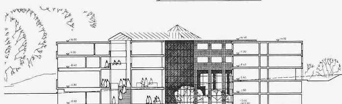
Coupe B-B
