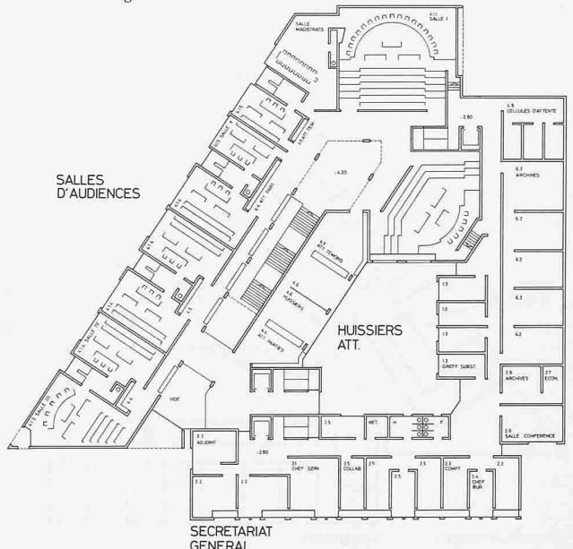
Plan du 1er étage
