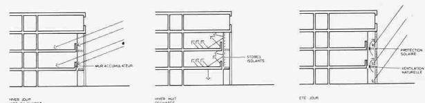
Coupe C-C, captage passif
