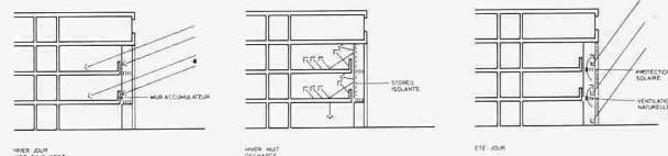
Coupe C-C, captage passif
