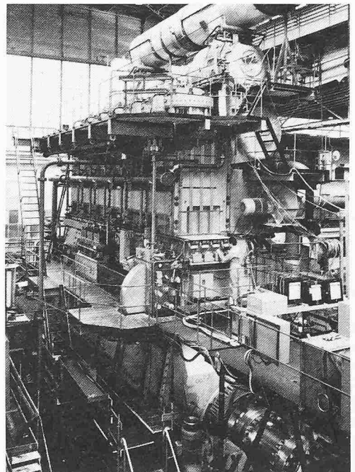
Ein Sulzer-Sechszylinder-RLA90-Motor auf dem Prüfstand in Winterthur
