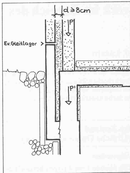
Skizze 6. Neue Detaillösung mit verbessertem Wärmeschutz bei hochliegendem Terrain
