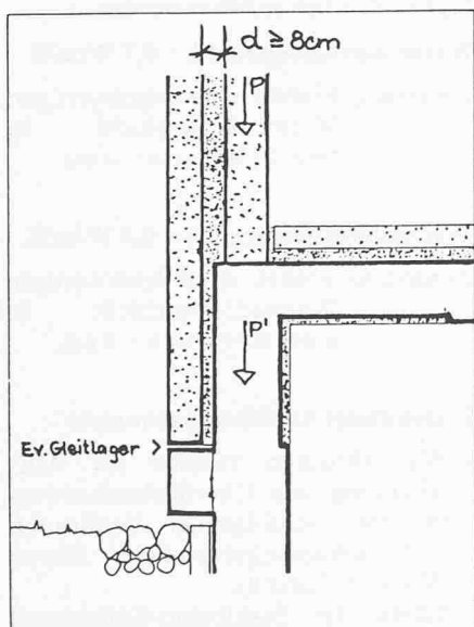
Skizze 5. Neue Detaillösung mit verbessertem Wärmeschutz bei tiefliegendem Terrain
