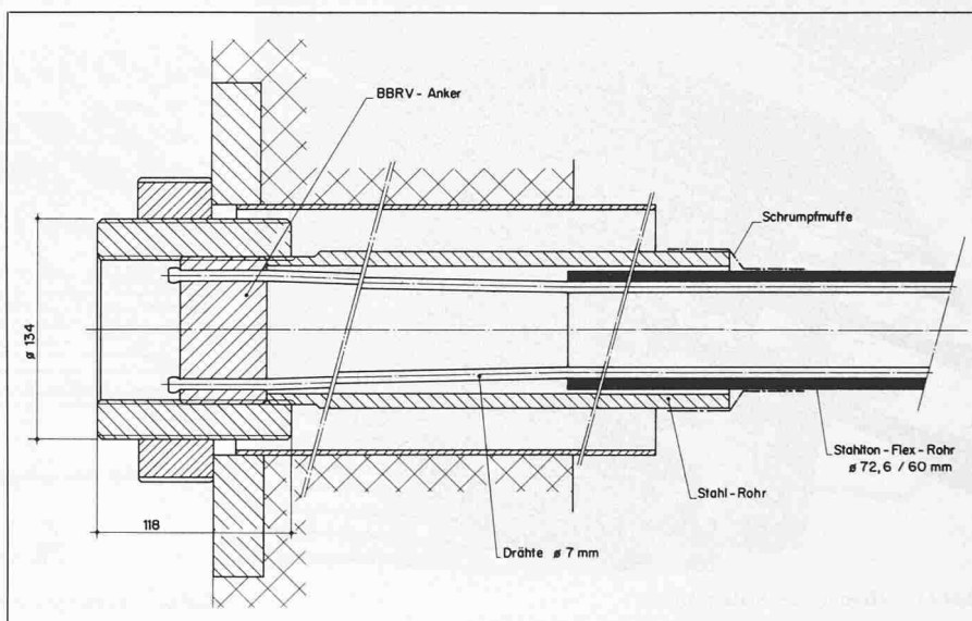
Bild 10. Paralleldrahtbündel für die Seilnetzkonstruktion, Detail der Verankerung
