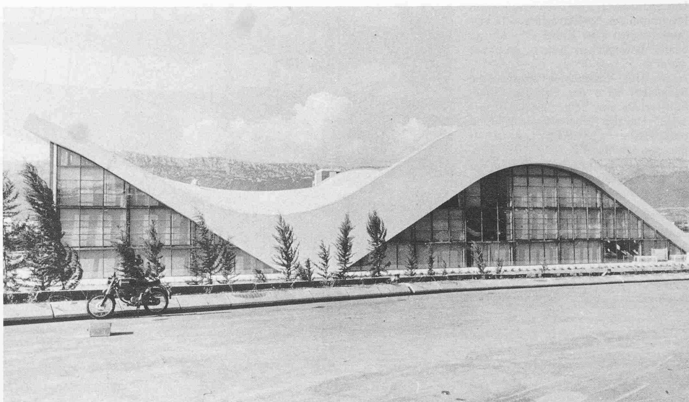
Bild 7. Schwimmhalle Split, Gesamtansicht
