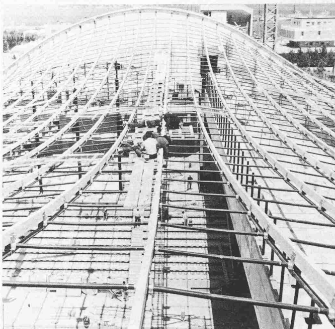
Bild 14. Montage der Auflagerkonstruktion auf das gespannte Seilnetz
