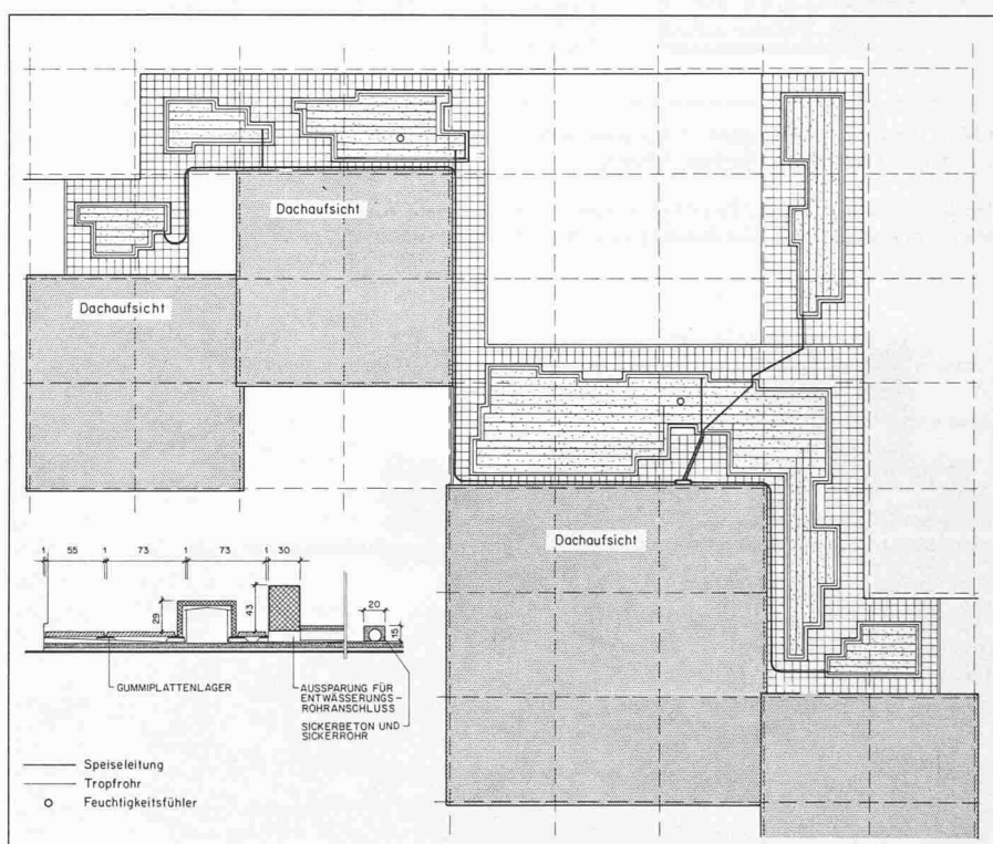
Bild 1. Grundrissausschnitt
