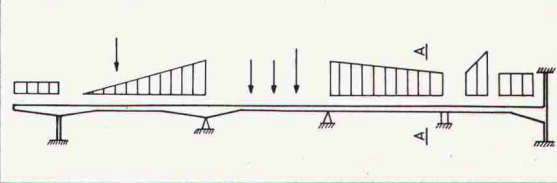
Programmsystem Grundbau
