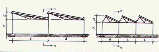
Programmsystem Bemessung
