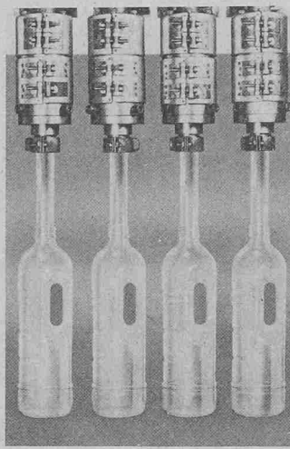
PVC-Getränkeflaschen mit Griff, auf der Bell-Blasformanlage gleichzeitig vierfach hergestellt.
