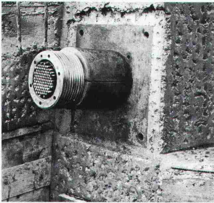
Brückenträger mit beweglicher Verankerung Typ M 4600
