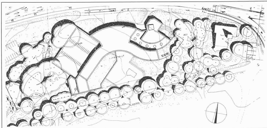
Lageplan 1:2400
