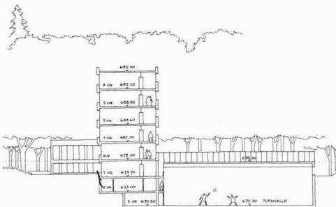
Schnitt Schule - Saal 1:1000
