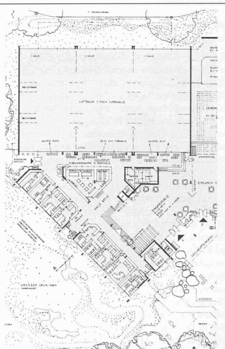
Grundriss Erdgeschoss B 1:1000
