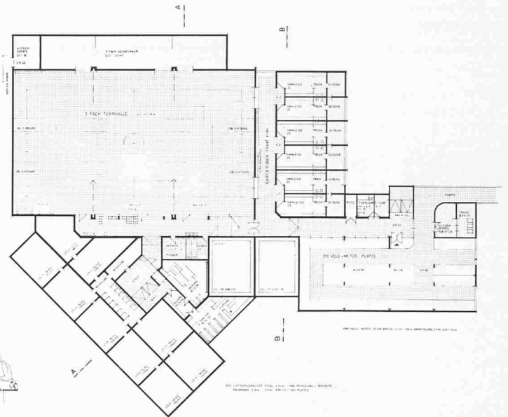
Grundriss Untergeschoss 1:1000
