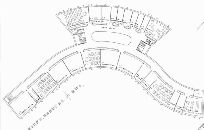
Grundriss 4. Obergeschoss 1:1000
