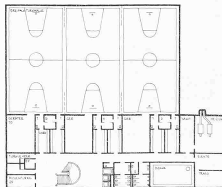
Oben: Grundriss Untergeschoss 1:1000
