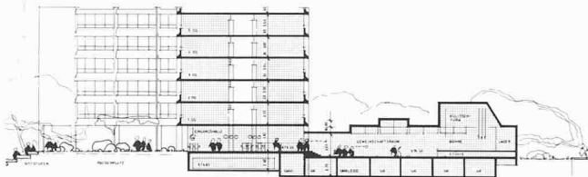
Schnitt B-B 1:1000
