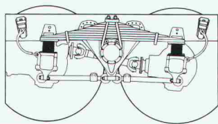
Erprobtes Volvo-Doppelachs-Aggregat mit progressiver Stahl-Gummifederung. Speziell geeignet für den harten Baustelleneinsatz.
