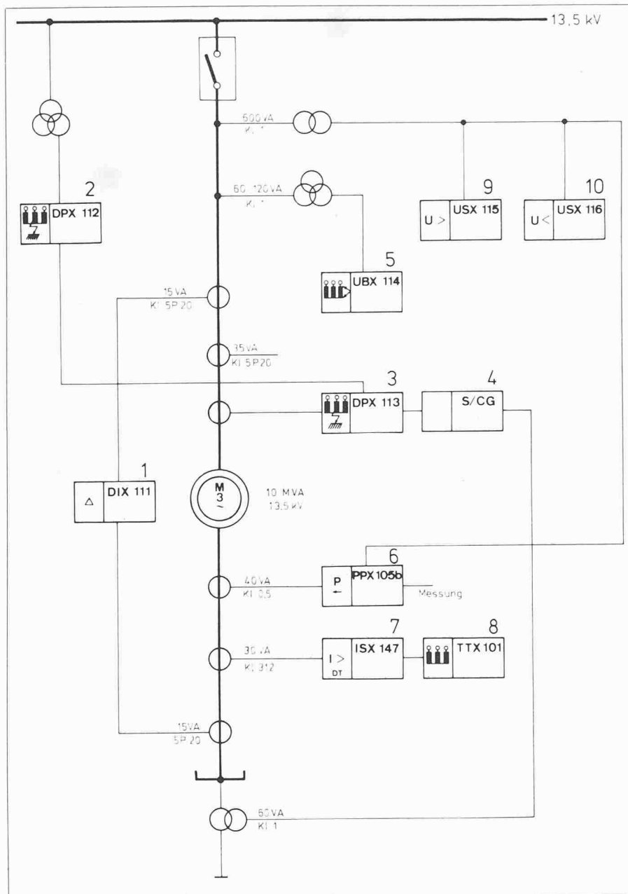
Bild 3. Generatorschutz-Relaisanordnung
