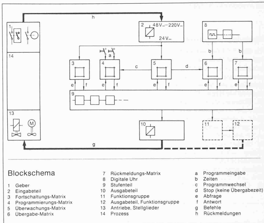
Bild 4. Blockschema der Folgesteuerungsautomatik «Secontic»
