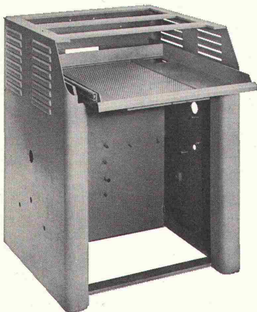
Metallkonstruktion
