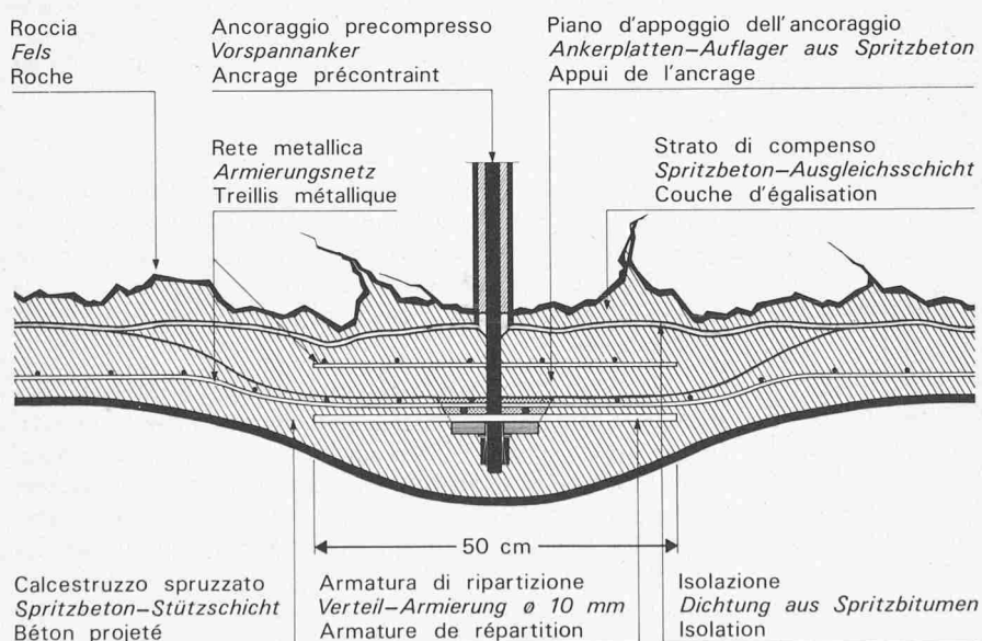
Bild 5. Verdrängende Isolation aus Spritzbitumen mit Schutz- und Stüttschicht aus Spritzbeton, Konstruktion im Bereich eines Ankerkopfes
