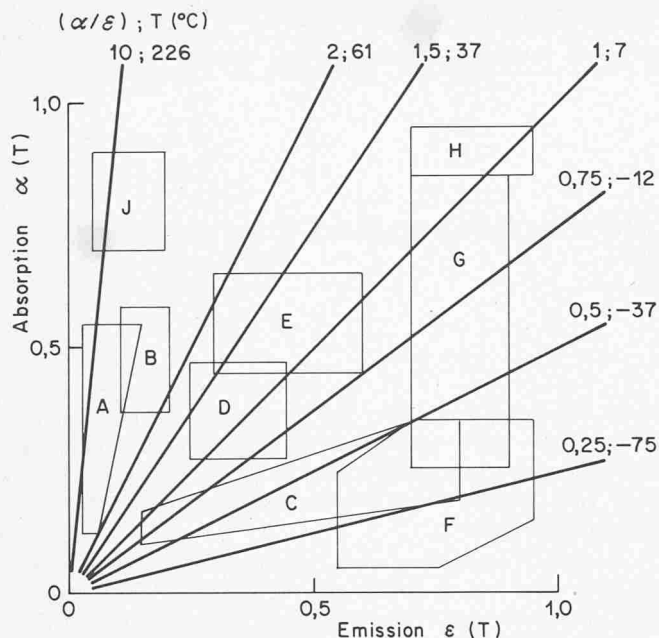
Bild 2. Einfluss des Verhältnisses (\alpha/\varepsilon) auf die Gleichgewichtstemperatur T(^{\circ}\text{C}) einer Kugel im Vakuum, die mit der Solarkonstanten beschienen wird. Charakterisierung verschiedener Oberflächenarten. A polierte Metalle B Metalle C bedampfte Metalle D metallische Farben E sandgestrahlte Metalle F weisse Farben, metallisierte Kunststoffe G diverse Farben H schwarze Farben J selektive Solarabsorber
