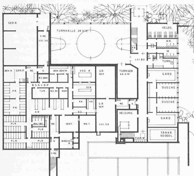
Grundriss Untergeschoss 1:650
