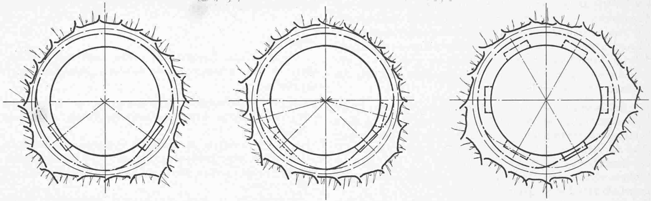
Bild 14. Mögliche «praxisgerechte» Anordnung der Verankerungsnischen innerhalb einer Gruppe benachbarter Kabel (Druckstollen)
