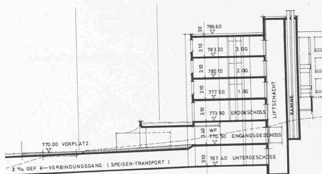
Unten: Schnitt durch Verbindungsgang zur bestehenden Küche 1:500
