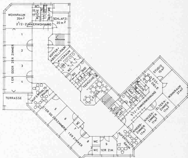
Grundriss 3. Obergeschoss 1:500, Vorschlag Personalunterkünfte
