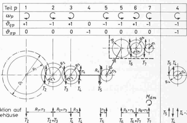
Bild 21. Kräfteverhältnisse in einem Kardanwellenantrieb mit querliegenden Kardanwelle und mit Quermotor
