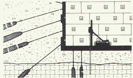
Fels- und Alluvial-Vorspannanker für Hang-, Fels- und Baugrubensicherung mehrfach korrosionsgeschützte Permanentanker Auftriebsanker, Tunnelverankerungen.
