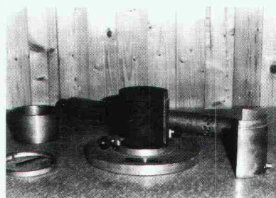
Verdichtungsversuch im Feldlabor
