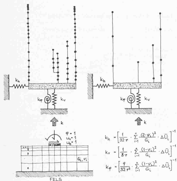
Bild 7. Balken-Federn-Modell des Projektverfassers (links) und des Prüfingenieurs (rechts)
