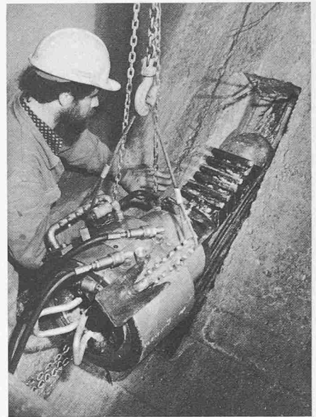
Fig. 7. Mise en tension des câbles Stressing of the cables
