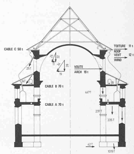
Fig. 3b. Coupe transversale de la nef Cross-section of the aisle
