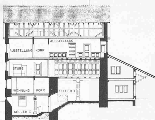
Rechts: Längsschnitt durch Burg und Anbau 1:350, Querschnitt durch Burg mit rückwärtigem Treppenhaus 1:350
