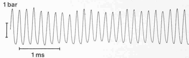
Bild 5. Zeitaufgelöstes Drucksignal, das in der Anordnung nach Bild 4 an der angedeuteten Stelle gemessen wurde. Es treten periodische Druckschwankungen mit sehr hoher Amplitude auf ( p_0/5 Spitze). Die Frequenz ist umgekehrt proportional zur Grösse der Anordnung. Der gemessene Verlauf mit einer Frequenz von 5600 Hz wurde für eine maximale Ausdehnung der Kavität quer zur Strömungsrichtung von 30 mm gewonnen
