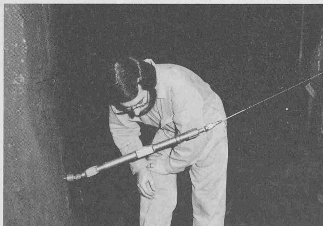
Präzisions-Längenmessgerät Distometer ISETH.
