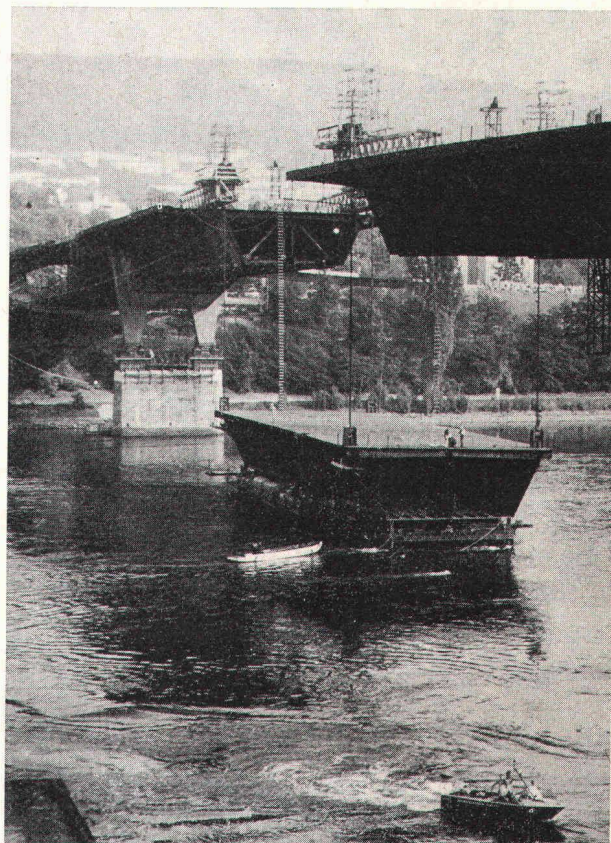
Hochheben des 650 Mp schweren Mittelteils der Horchheimer Rheinbrücke bei Koblenz.
