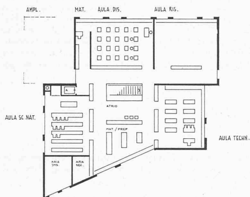
Grundriss 1. Obergeschoss 1:600
