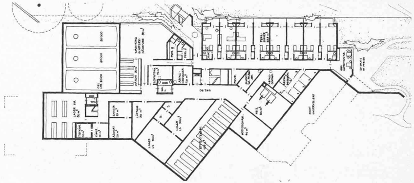
Grundriss Untergeschoss 1:800
