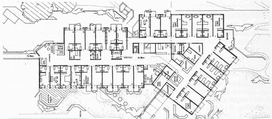
Grundriss 1. Obergeschoss 1:800
