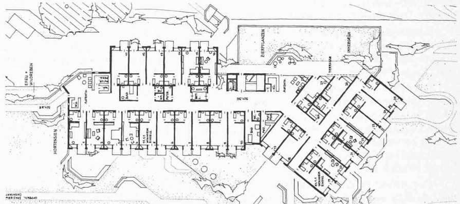
Grundriss 2. Obergeschoss 1:800
