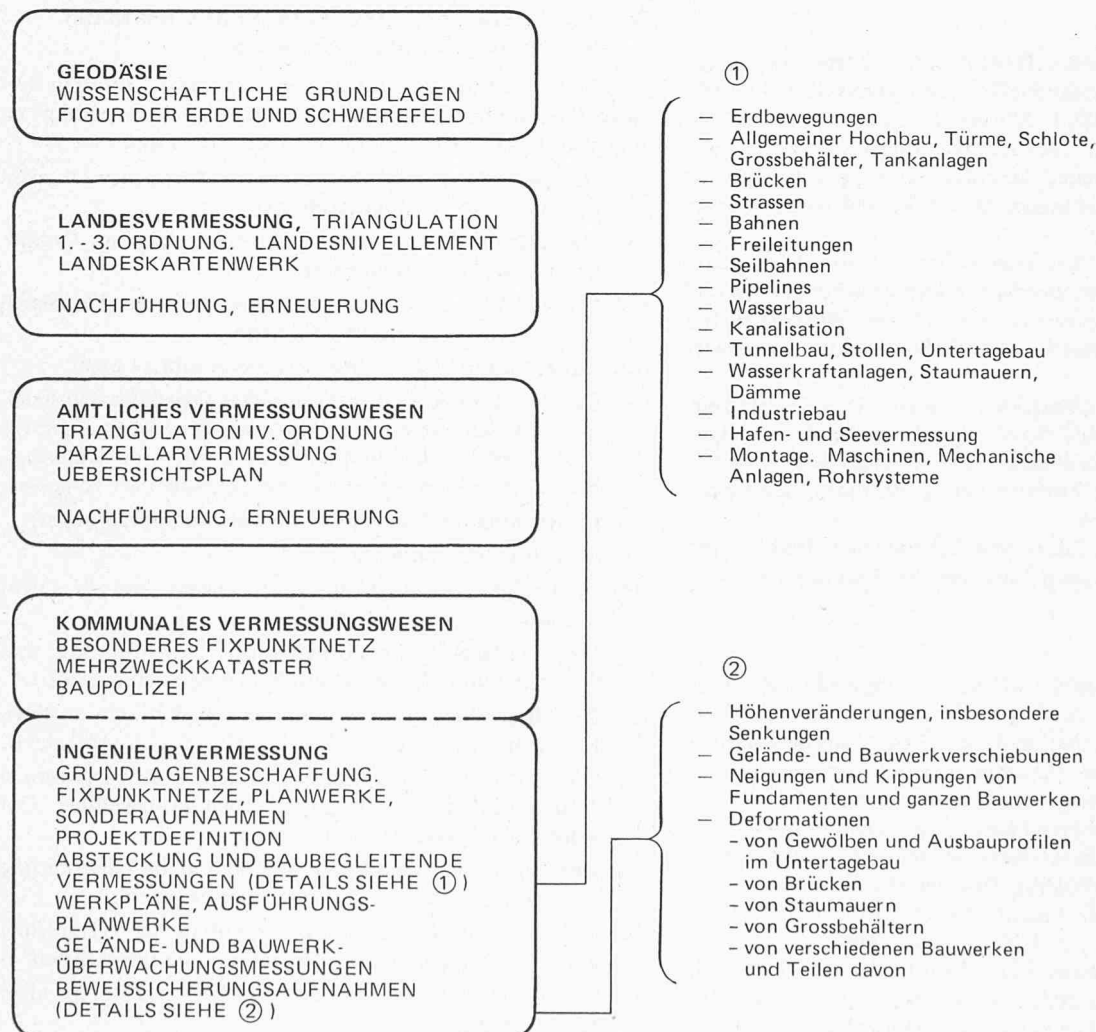
Tafel 1. Gliederung des Vermessungswesens
