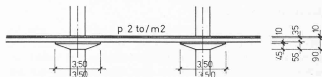
VARIANTE PILZDECKE
