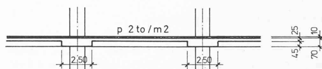
AUSGEFÜHRTE KASSETTENDECKE
