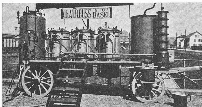
Bild 3. Fahrenbare Obstsaft-Eindampfanlage mit Brüdenverdichtung aus dem Jahre 1933
