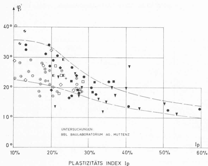
Bild 9. Scherwinkel in Funktion des Plastizitätsindex I_p
