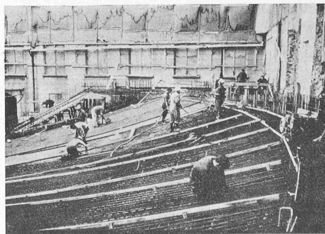
Bild 3. Auditoriumsschale im Bauzustand
