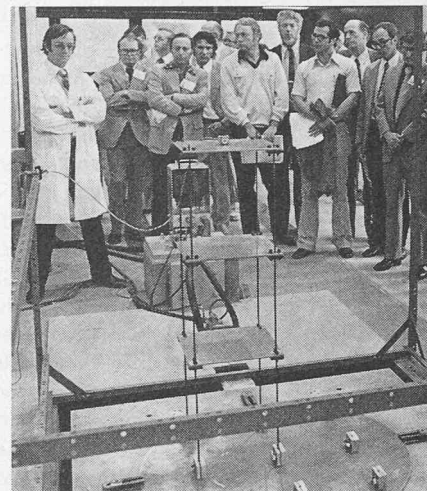
Teilnehmer an der Eröffnungsfeier im Labor für dynamische Testversuche. Gezeigt wird das Modell eines dreistöckigen Gebäudes auf dem Schütteltisch
